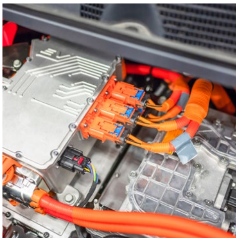
Kennzeichnung der HV-Leitungen in Signalfarbe orange / Marking of the HV-Lines in signal color orange
